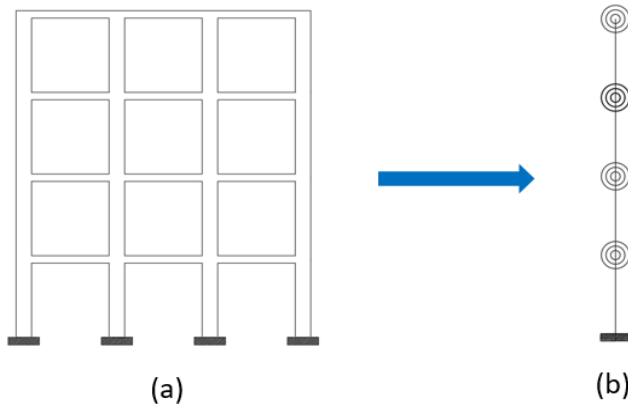
Şekil 4. (a) Ayrıntılı sonlu eleman modeli (b) Kirişsiz Fishbone modeli
