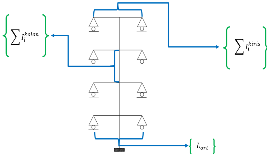
Şekil 2. Geleneksel Fishbone modelinde eşdeğer kolon ve eşdeğer kirişlerin hesaplama ve konumlandırma ayrıntıları
