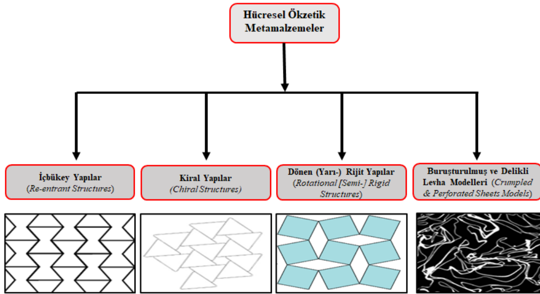
Şekil 2. Hüresel ökzetik yapıların genel sınıflandırması (Kelkar ve ark. (2020) tarafından sunulan bilgilerden uyarlanmıştır).
