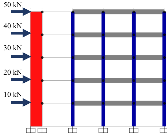
Şekil 3. Perde-Çerçeve sistem modeli
