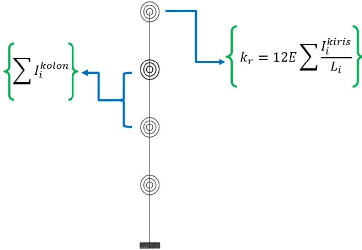
Şekil 5. Kirişsiz Fishbone modelinde eşdeğer kolon ve dönel yayların hesaplanması ve konumlandırma ayrıntıları
