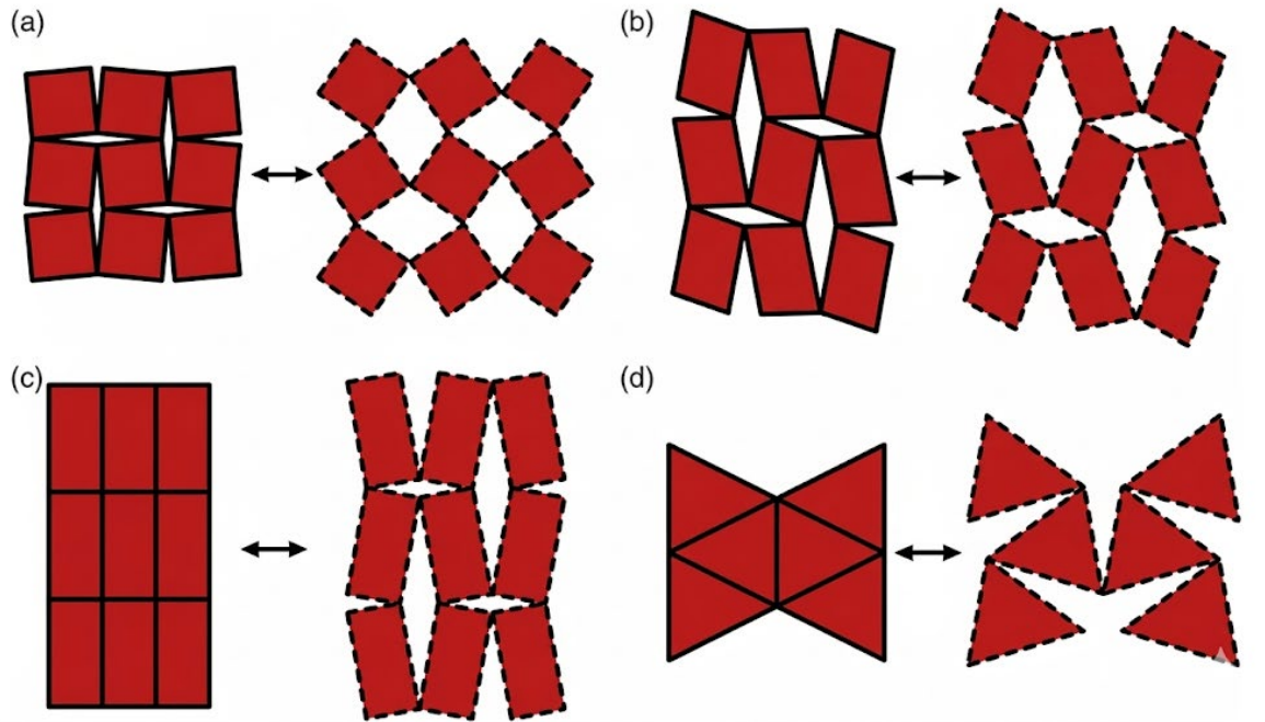
Şekil 6. Farklı geometrilere sahip dönen rijit yapılar (Wang vd., 2020 tarafından sunulan bilgilerden uyarlanmıştır).
