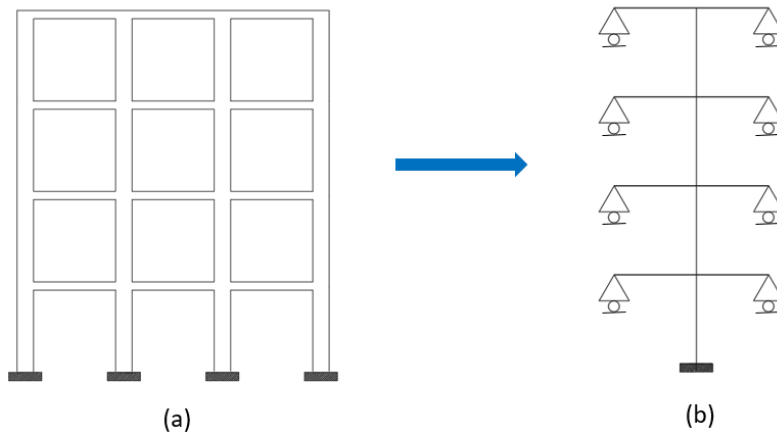
Şekil 1. (a) Ayrıntılı sonlu eleman modeli (b) Geleneksel Fishbone modeli
