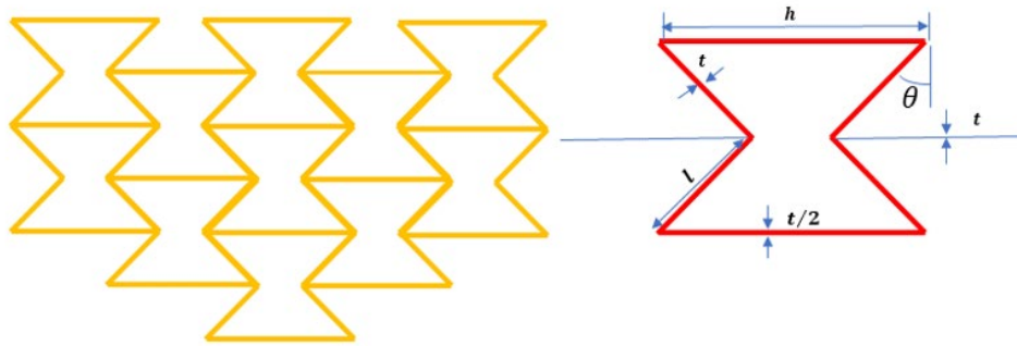
Şekil 3. Re-entrant (içbükey) bal peteği yapısı (Wang vd., 2019 tarafından sunulan bilgilerden uyarlanmıştır).
