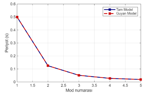
Şekil 4. Tam model ile Guyan indirgenmiş modelin grafiksel karşılaştırması a) yatay ötelenme, b) doğal titreşim periyodu
