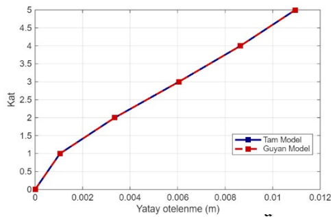
Şekil 4. Tam model ile Guyan indirgenmiş modelin grafiksel karşılaştırması a) yatay ötelenme, b) doğal titreşim periyodu
