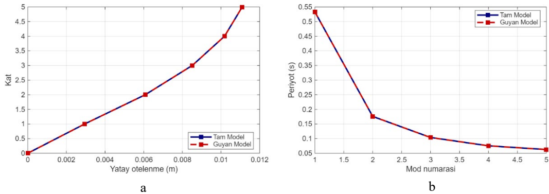
Şekil 2. Tam model ile Guyan indirgenmiş modelin grafiksel karşılaştırılması a) yatay ötelenme, b) doğal titreşim periyodu
