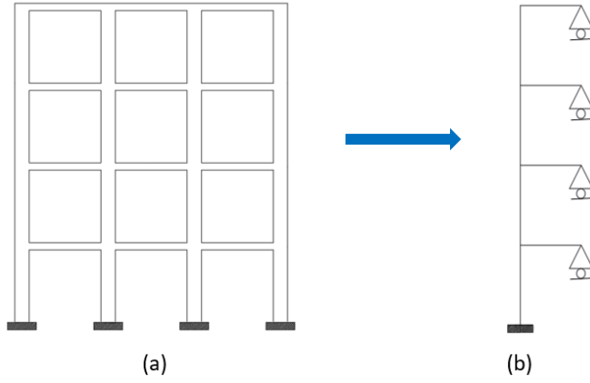
Şekil 3. (a) Ayrıntılı sonlu eleman modeli (b) Light-Foot modeli
