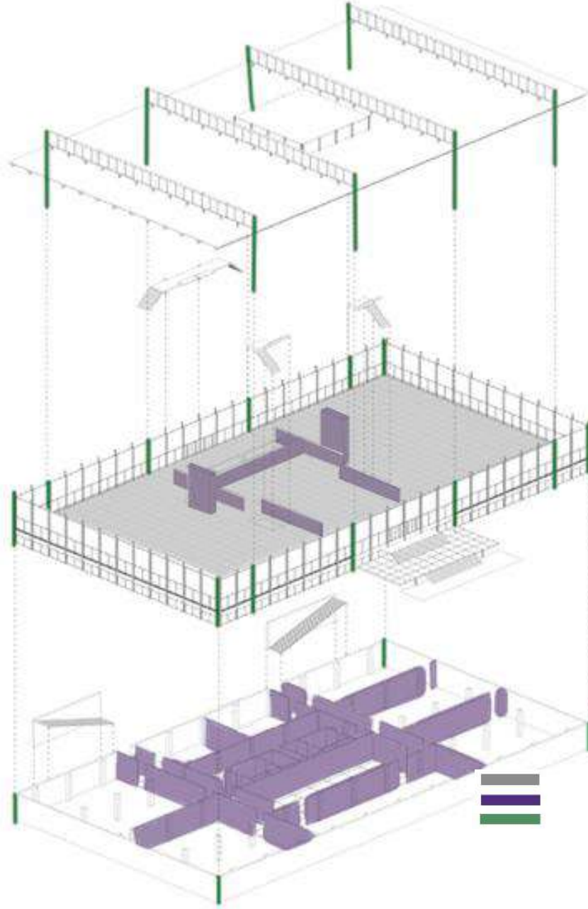
řekil 3. IIT Crown Hall plan diyagramı (miessociety.org dan alınıp iřlenmiřtir)
