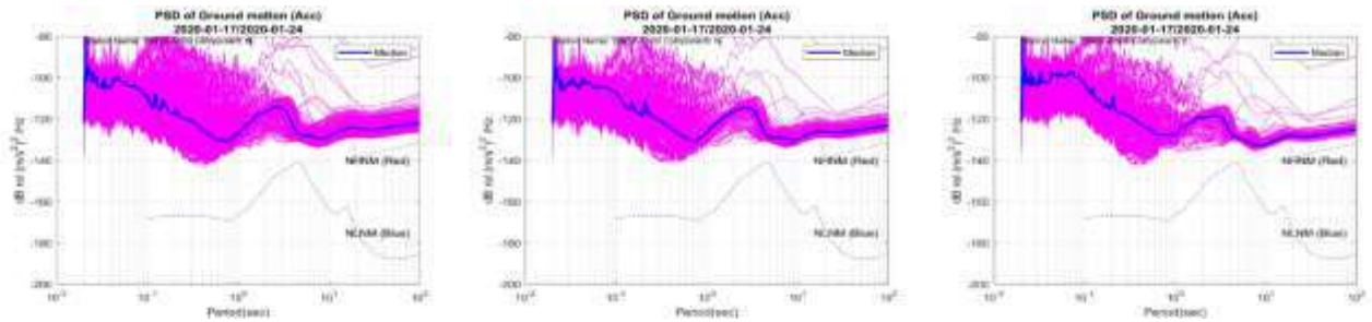
Şekil 3. AYVC (Ayvacık) istasyonu Z, N-S ve E-W bileşenleri 1 aylık Güç Spektrumu Yoğunluğu grafikleri (Yer: Ayvacık Belediyesi binası zemin kat, jeoloji: Volkanik).
