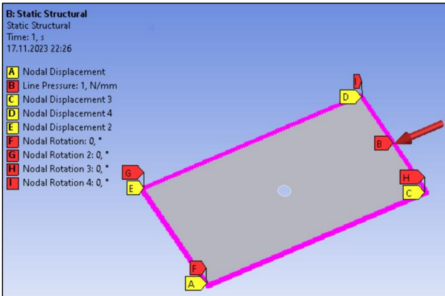
Şekil 2. Ansys sonlu elemanlar yazılımı sınır şartları.
