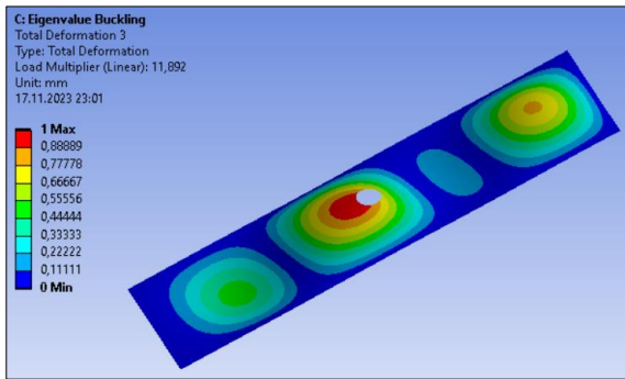
c) Eigenvalue buckling mod 3.
