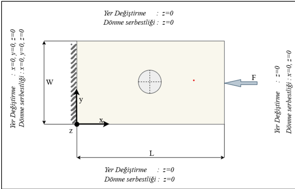
Şekil 1. Delikli kompozit plakanın boyutsal tanımlanması ve sınır şartları.
