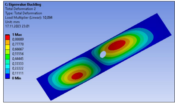
b) Eigenvalue buckling mod 2.
