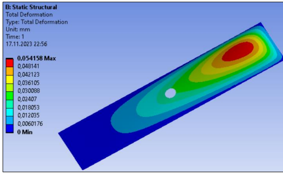
a) Total deformasyon.
