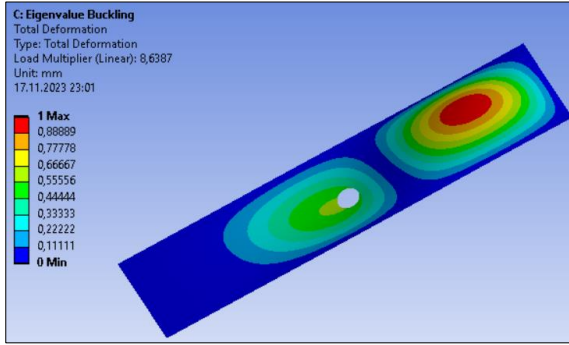
a) Eigenvalue buckling mod 1.
