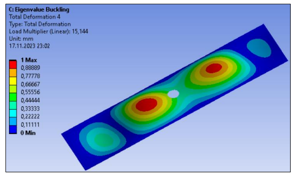
d) Eigenvalue buckling mod 4.
