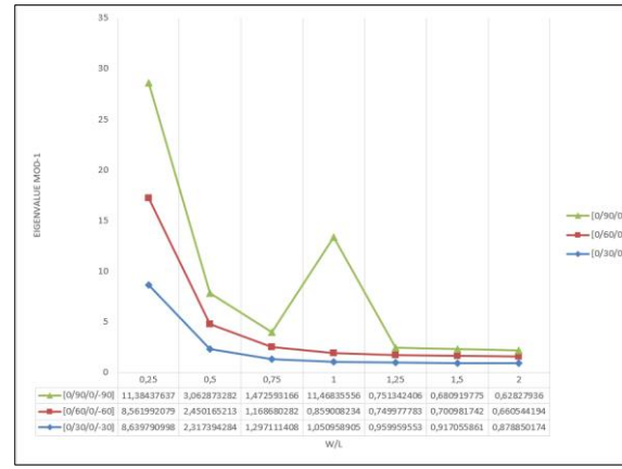
b) Katman açısı en-boy oranı karşılaştırması.
